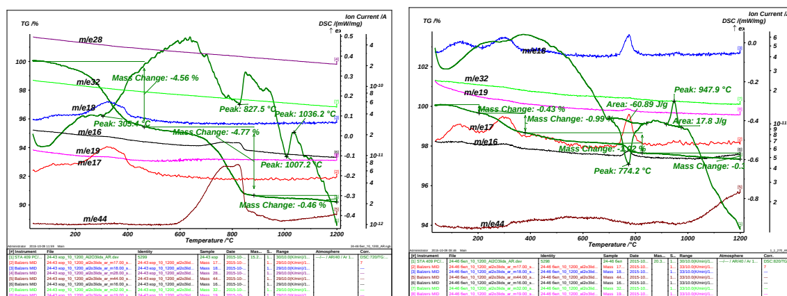
Спектры ДСК-ТГ коричневого и асбест-чароита при нагревании
