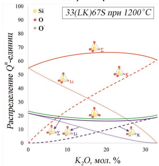
Рис. 1. Распределение структурных единиц в расплаве состава 33(\text{Li}_2\text{O}+\text{K}_2\text{O})\text{SiO}_2 при 1200^\circ\text{C} .
