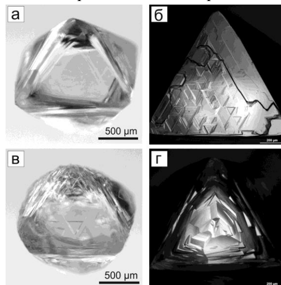
Рис. 1. Общий вид кристалла природного алмаза и микрорельеф его граней {111} до (а-б) и после (в-г) эксперимента при 1300°C.
