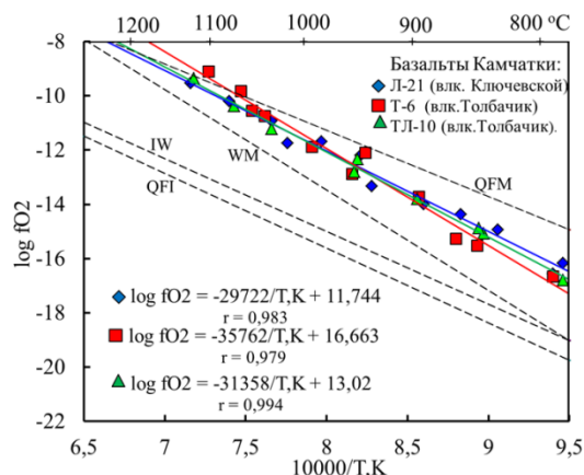
Рис. 1. Зависимость \log fO_2 vs T, K для базальтов Камчатки.
