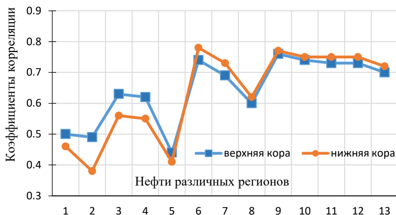
Рис. 1. Изменение корреляции между МЭ составом нефтей различных НГБ и усредненным составом верхней и нижней континентальной коры
